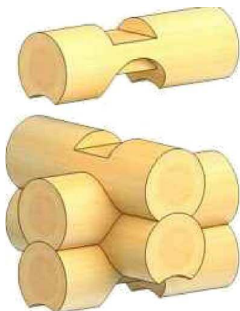
1. spôsob zrubovej väzby guľatiny
