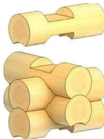
2. spôsob zrubovej väzby guľatiny
